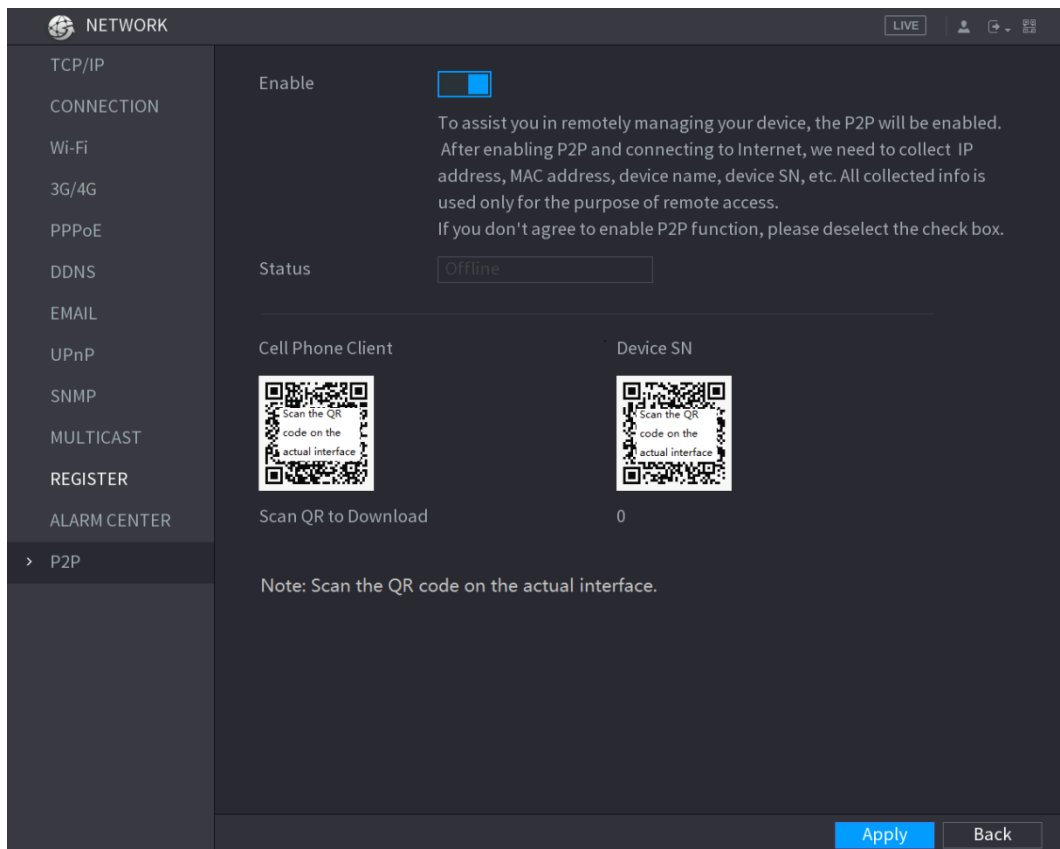
Rysunek 3-4 Interfejs P2P
