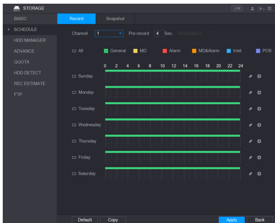
Rysunek 3-2 Konfiguracja harmonogramu nagrań
